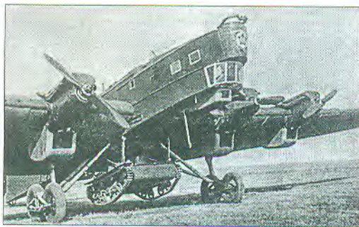
Легкий танк Т-38, закріплений під літаком ТБ-3 на підвісці ДПТ-2. Фото 1939 року
